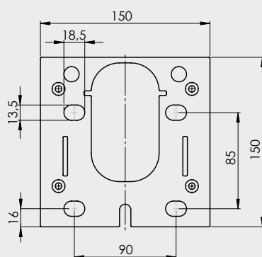
Golvplatta för stolpe
