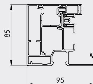
Sidoskena
