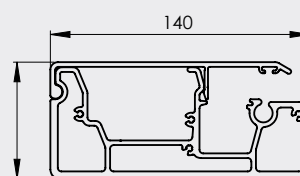
Enkelskena
