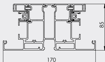
Dubbelskena
